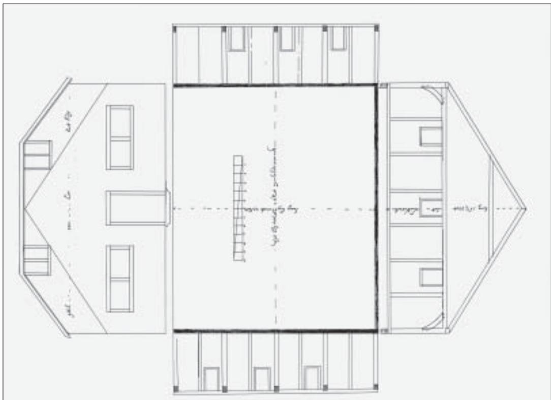
Bouwtekening voor de uitbreiding van de schuurkerk aan de Voorweg in 1768 (Algemeen Rijksarchief, Den Haag).
