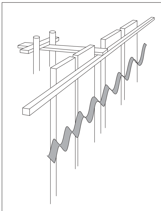
Schets van een beschoeiing met trekballenconstructie.
