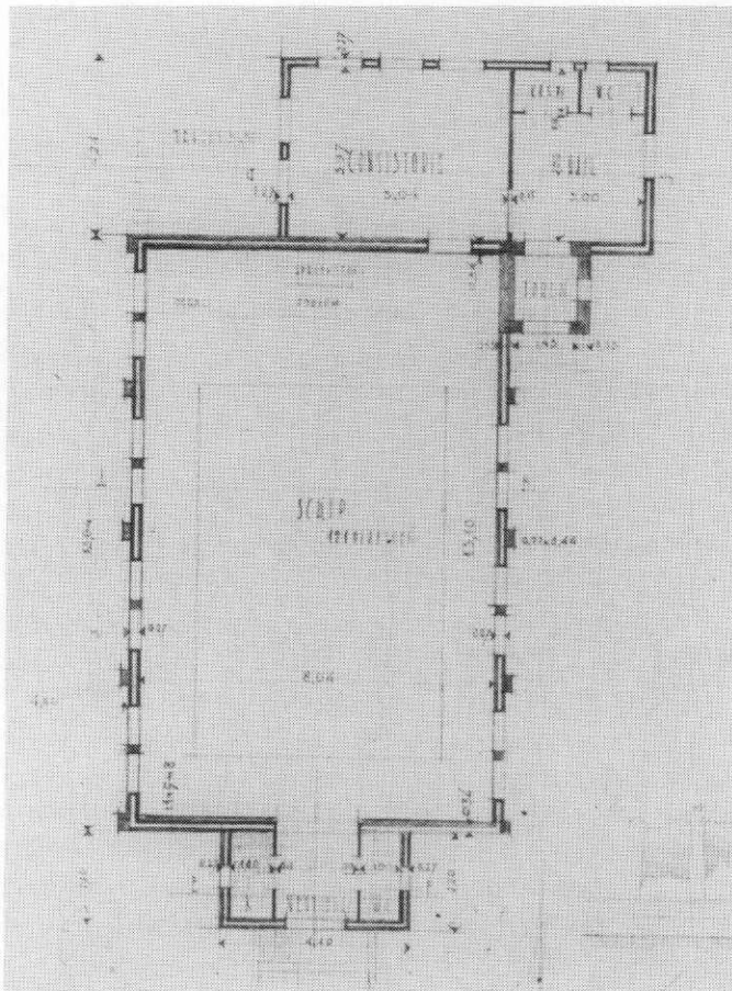
Afbeelding 20. Bouwtekening van de Adventskerk door A. van Eck, 1955.
