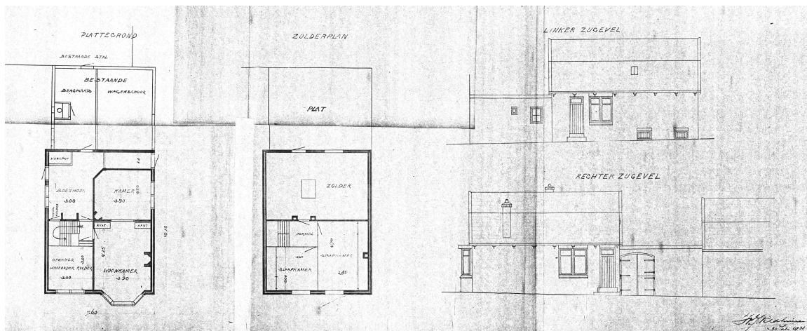
Voorweg 170 in 1931: plattegronden en zijgevels
