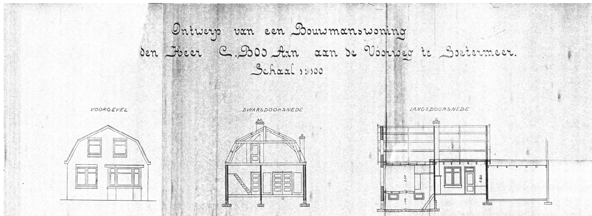
Voorweg 170 in 1931: voorgevel en doorsneden
