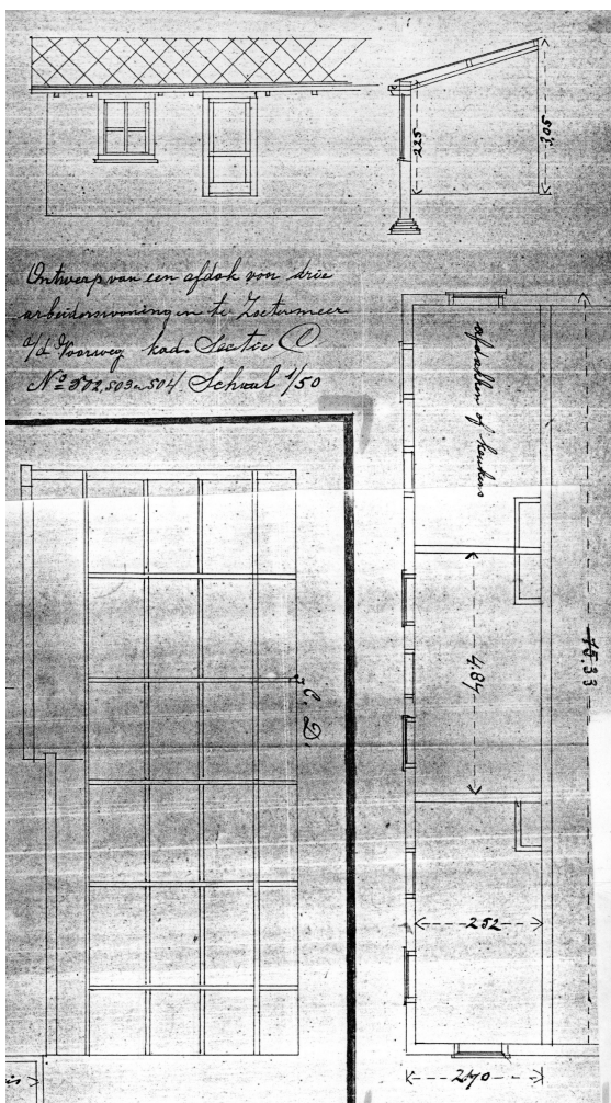
1914: vernieuwing van het afdak achter Voorweg 164-168; het linkerdeel van de tekening hoort bij een ander plan
