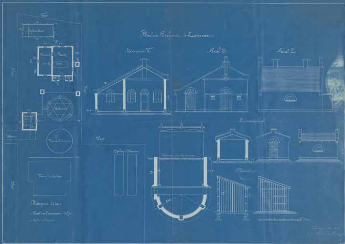
Ontwerptekening gasfabriek aan de Delftsewallen, 1907
