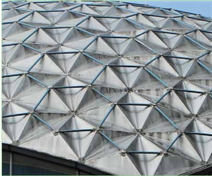
Koepелеlementen, een dubbellaags systeem: dak en detail (foto Dick Valentijn, bewerking Paul Schoenmakers)
